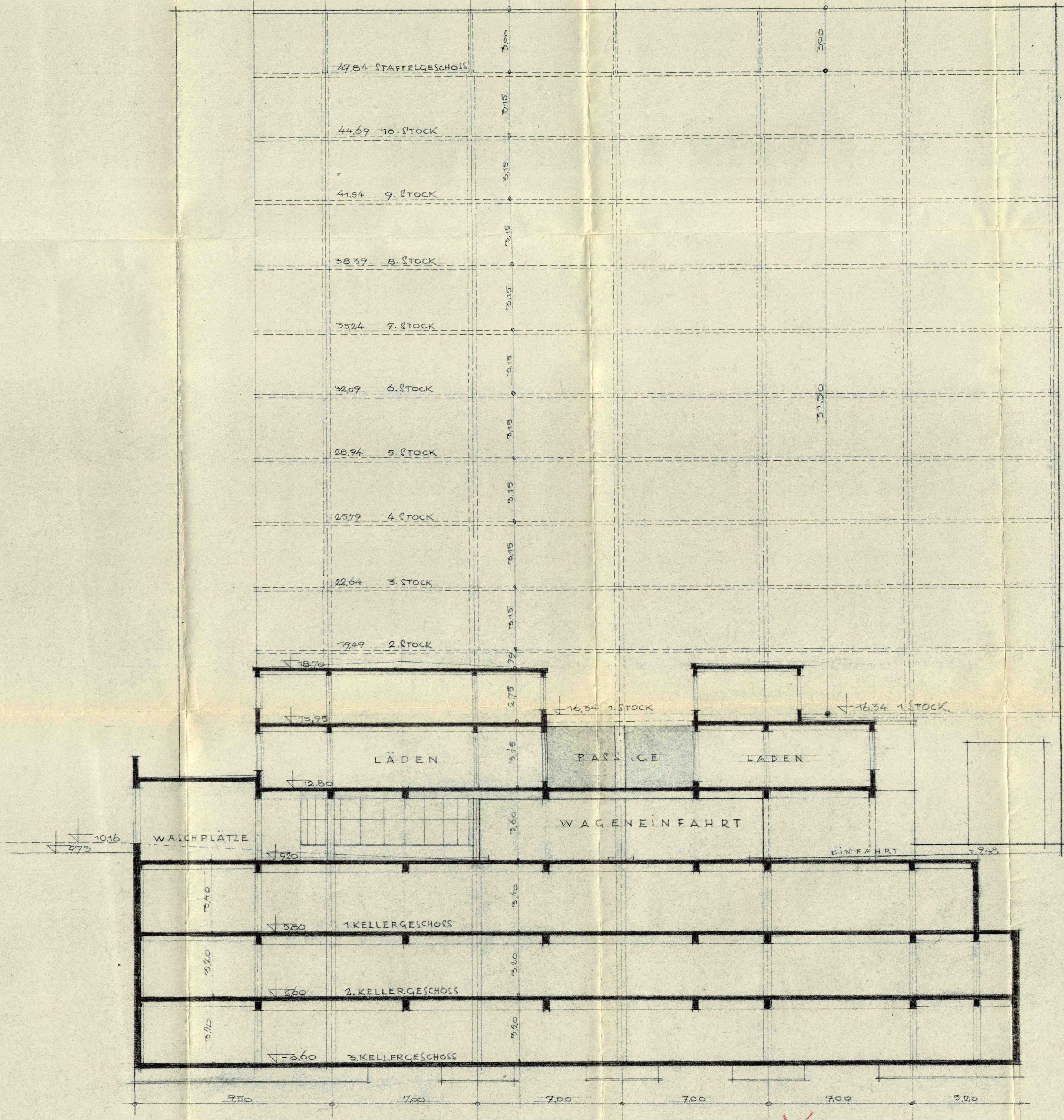
SCHNITT C - D · ZWISCHENBAU BLOCK D
