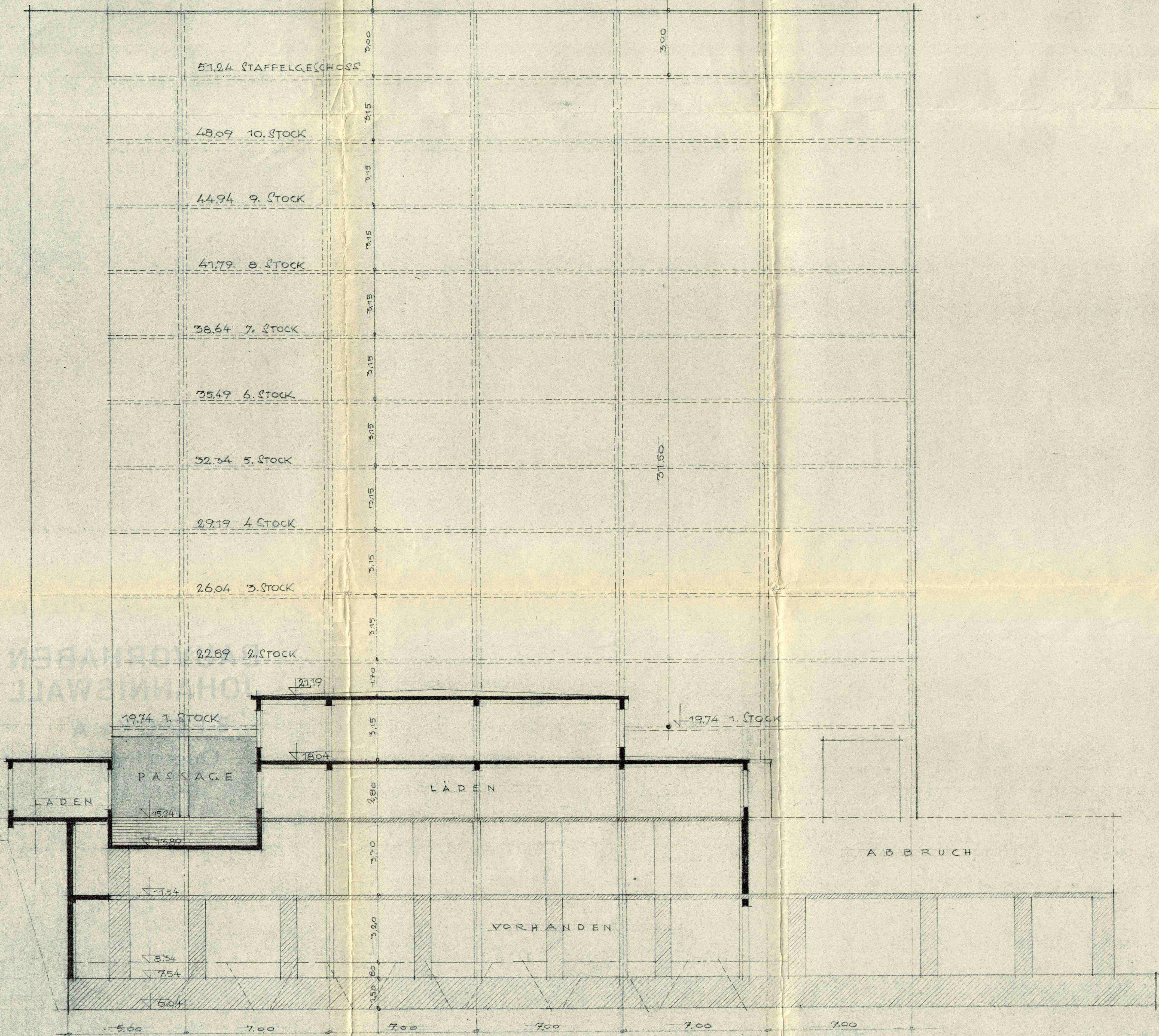
SCHNITT A - B · ZWISCHENBAU BLOCK A
